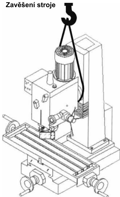
Zavěšení stroje
