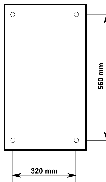
Rozteče děr základny frézky
